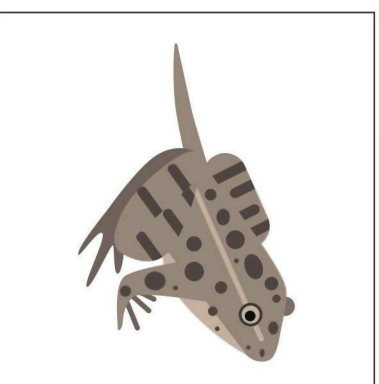
ХВОСТ УКОРАЧИВАЕТСЯ
